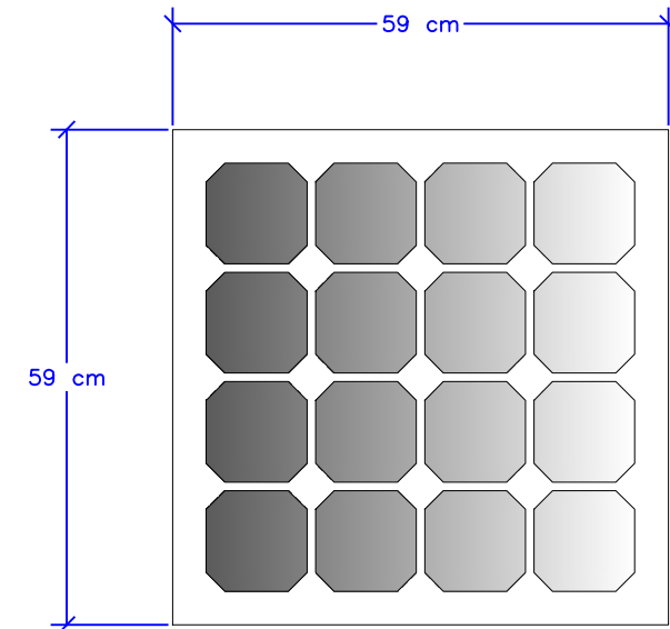
ALZADO LAMINADO FOTOVOLTAICO
